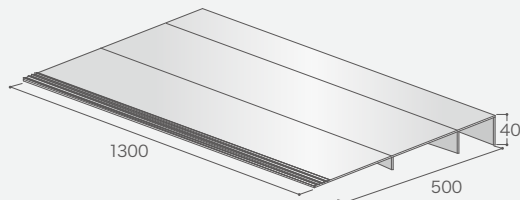
キヨレックススロープ H40 ロングタイプ (勾配 1/12.5)
