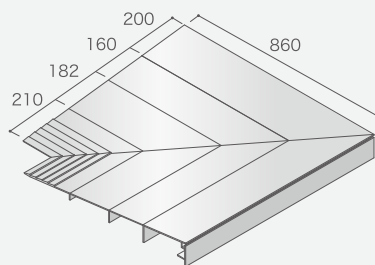
キヨレックススロープ入隅 H50, H70, H95
