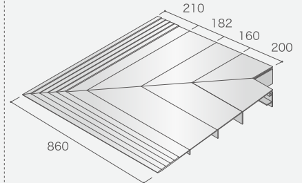
キヨレックススロープ出隅 H50, H70, H95
